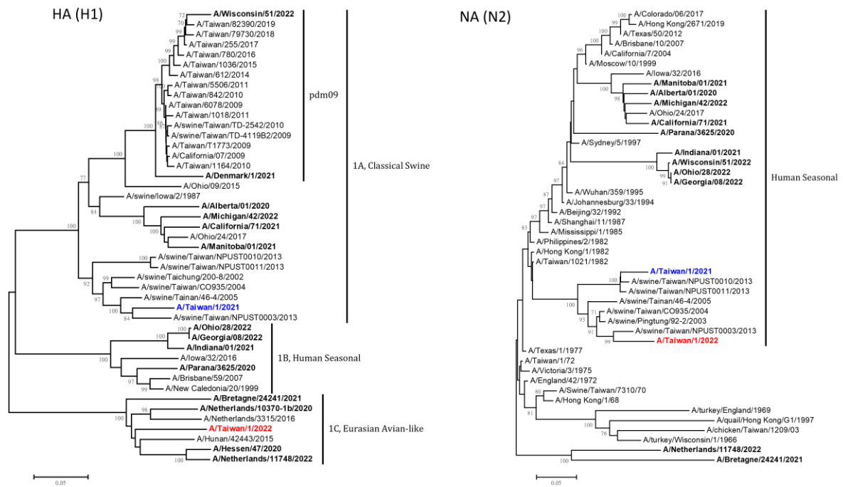
圖三、A/Taiwan/1/2022(H1N2)v HA 與 NA 親緣樹狀圖
