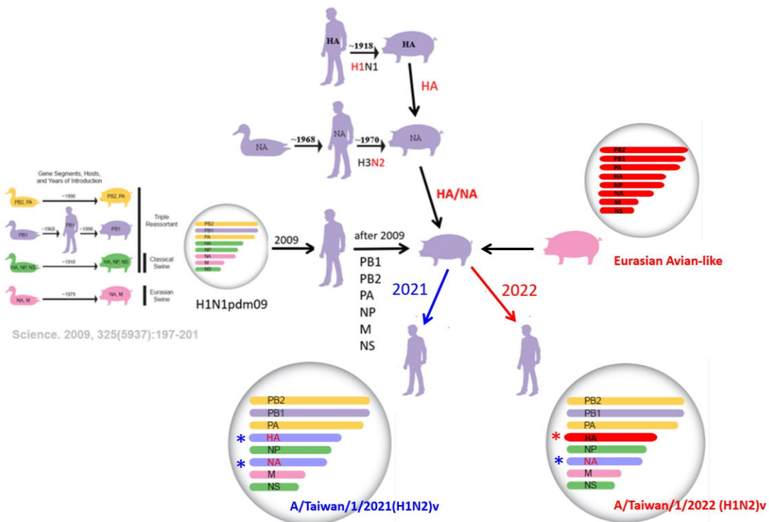
圖四、台灣人類 2022 與 2021 H1N2v 流感病毒 8 個基因片段之來源。
