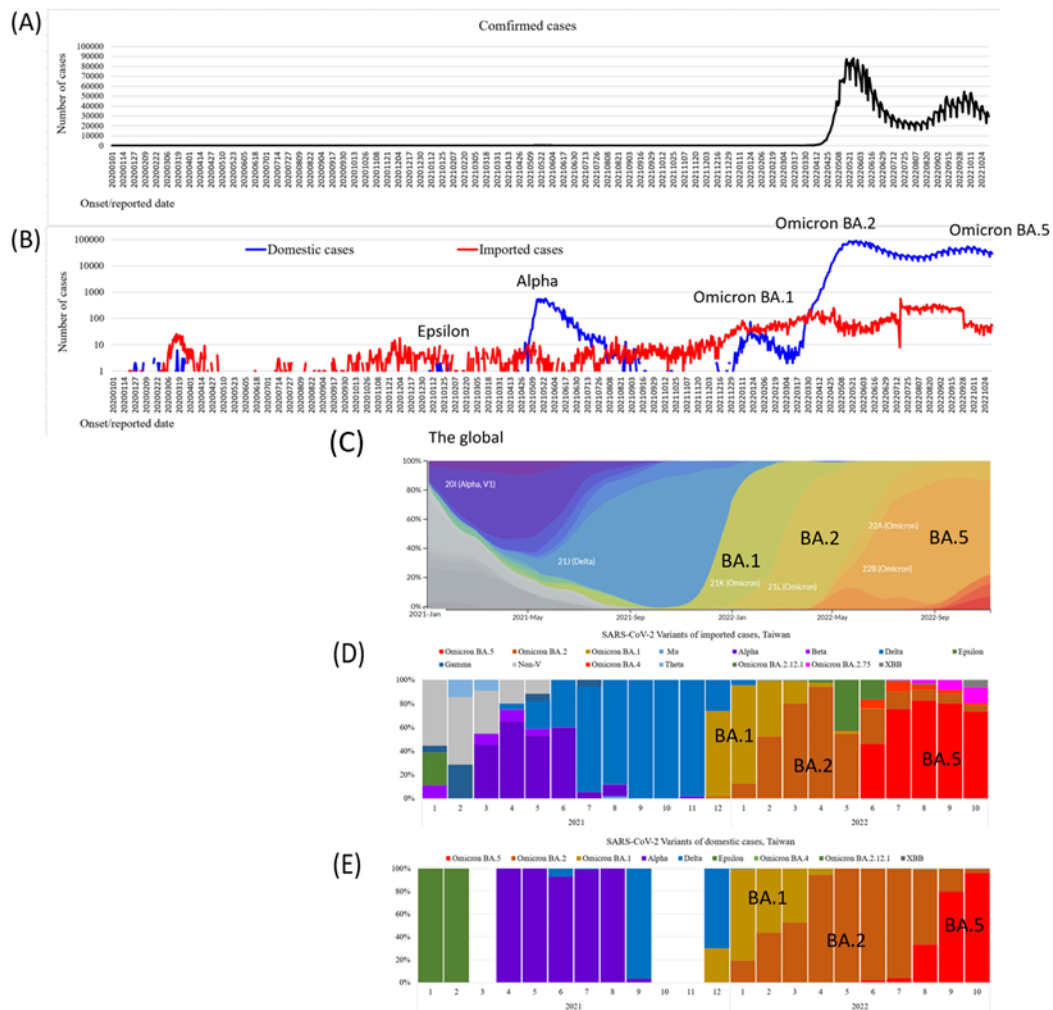
圖一、台灣 COVID-19 2020-2022 確診個案數目變化與病毒型別替換，(A)全部確診個案數目，(B)本土與境外確診個案數目，確診數目以指數呈現，(C)全球病毒型別，(D)境外確診個案病毒型別，(E) 本土確診個案病毒型別。
