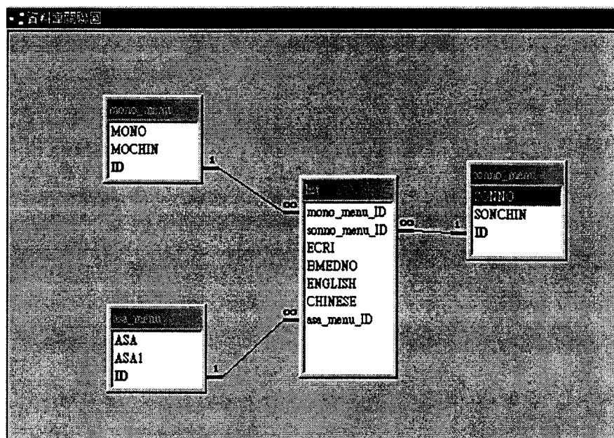
圖一、資料庫關聯圖
