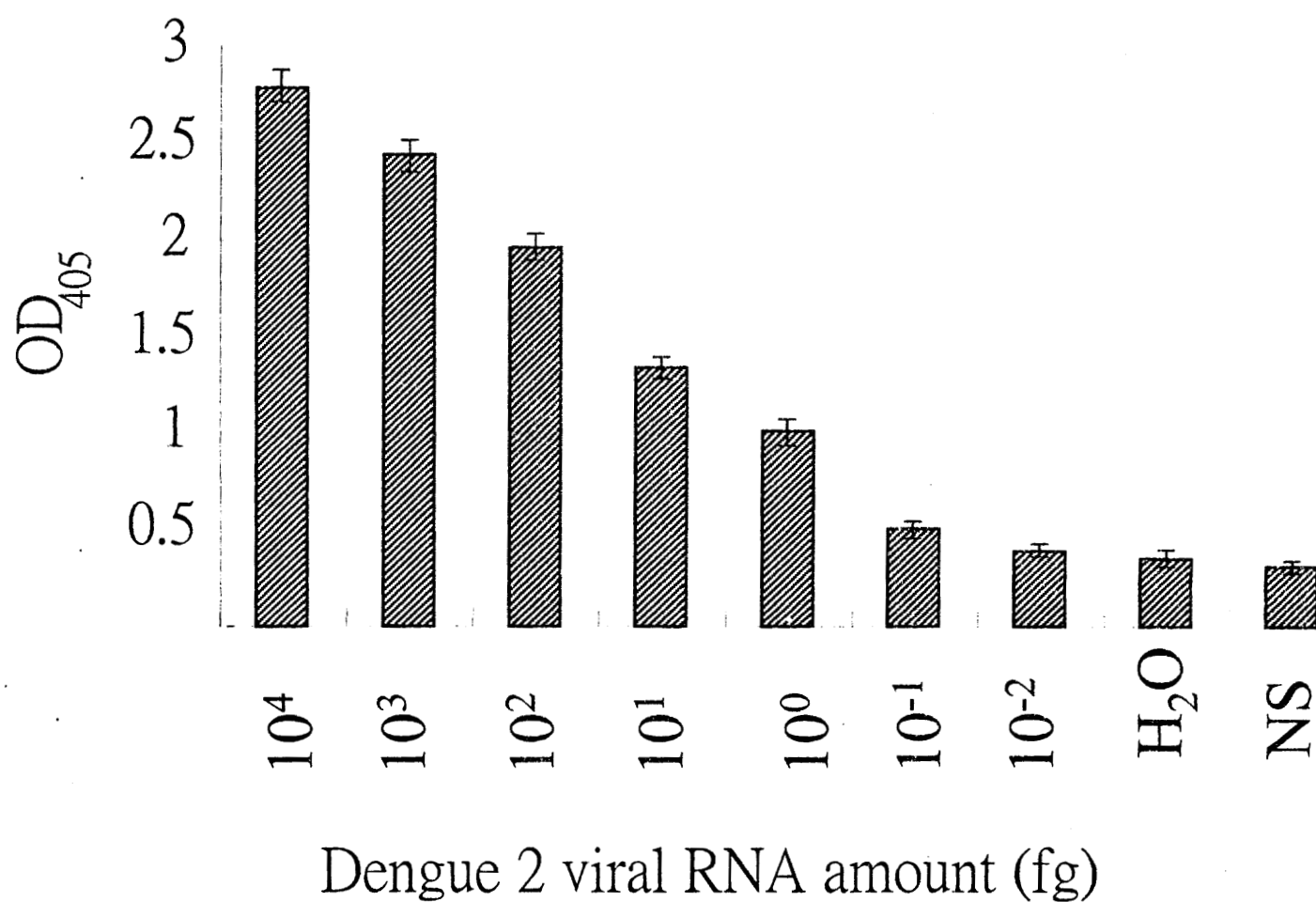
圖十：以 streptavidin coated plate based assay 檢測第二型登革病毒之靈敏度。病毒 RNA 以 fg 為單位， H_2O 為 negative control，NS 為登革病毒陰性血清檢體。
