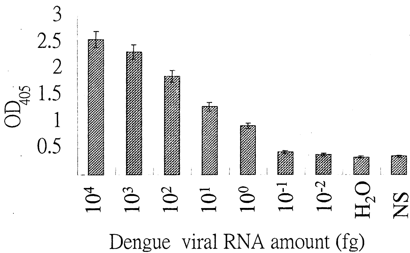
圖九：以 streptavidin coated plate based assay 檢測第一型登革病毒之靈敏度。病毒 RNA 以 fg 為單位，H 2 O 為 negative control，NS 為登革病毒陰性血清檢體。
